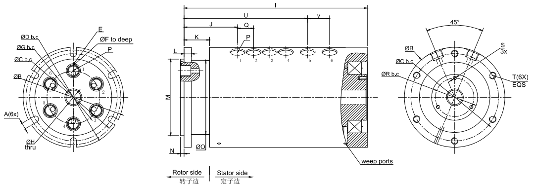
MGP6 (多功能旋转接头) 尺寸图
